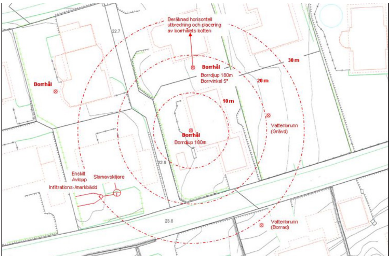
Figur 1. Exempelritning
