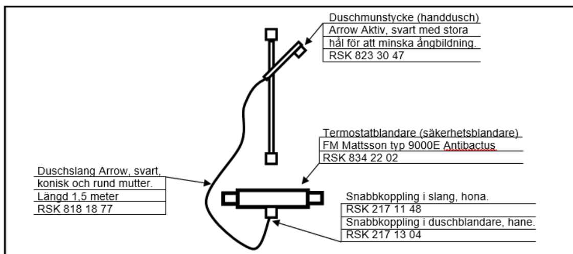
Figur 4. Princip och material för duschanordning och blandare i VoB.
