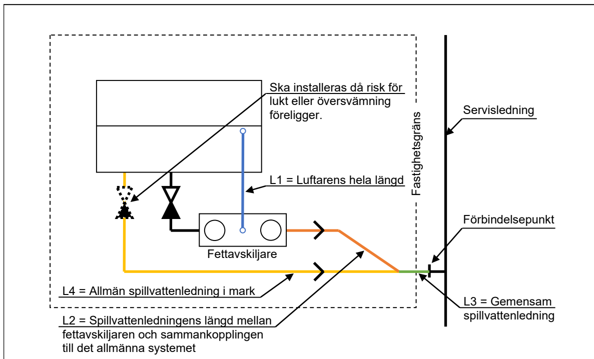
Figur 5. Princip spillvattensystem.
