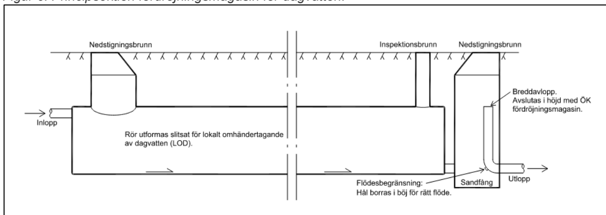
Figur 6. Principsektion fördröjningsmagasin för dagvatten.
