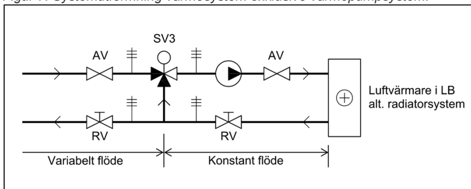
Figur 7. Systemutformning värmesystem exklusive värmepumpsystem.
