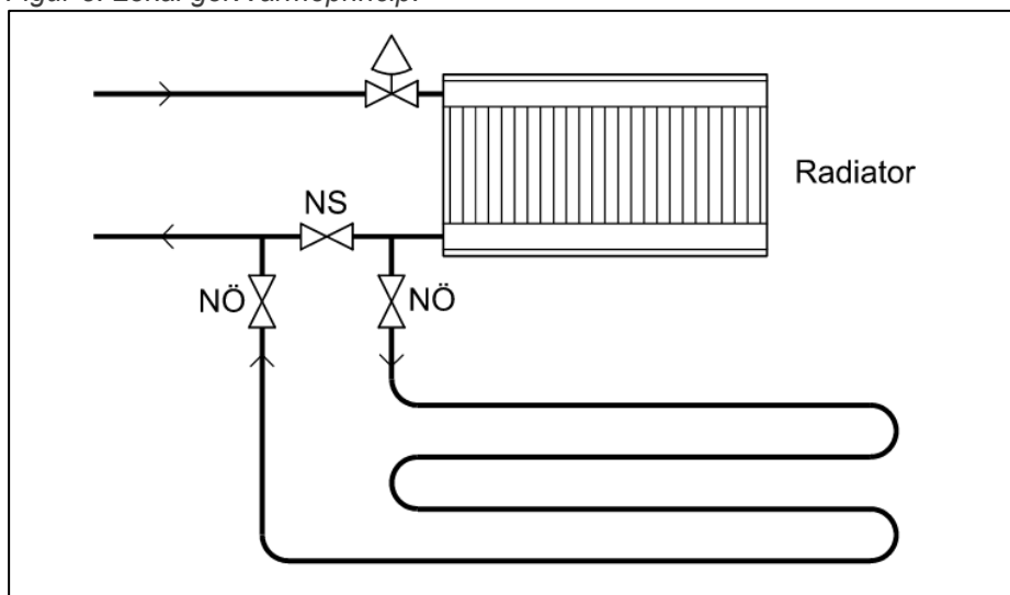
Figur 8. Lokal golvvärmeprincip.
