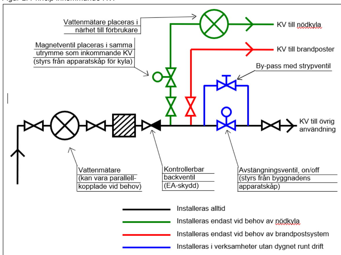
Figur 2. Princip inkommande KV.
