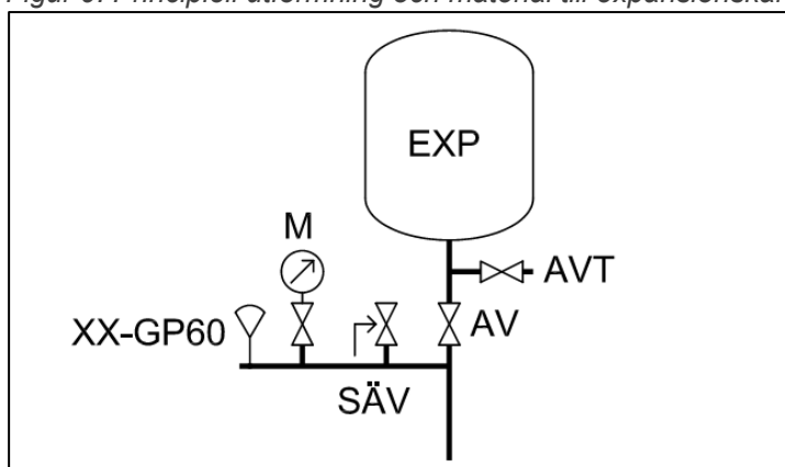
Figur 9. Principiell utformning och material till expansionskärl.
