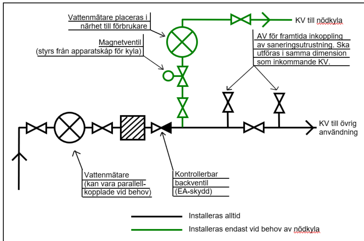
Figur 3. Princip inkommande KV VoB.
