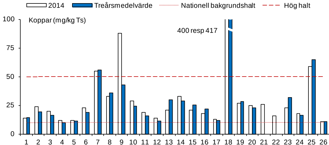
Figur 7. Halter av koppar vid samtliga undersökta lokaler 2014 samt beräknade treårsmedelvärden. Halter över 50 mg/kg Ts klassas som höga (streckad linje). Den prickade linjen anger nationell bakgrundshalt (10 mg/kg Ts).
