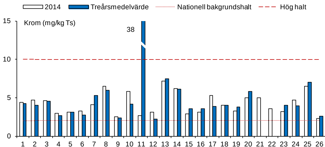
Figur 9. Halter av krom vid samtliga undersökta lokaler 2014 samt beräknade treårsmedelvärden. Halter över 10 mg/kg Ts klassas som höga (streckad linje). Den prickade linjen anger nationell bakgrundshalt (2 mg/kg Ts).
