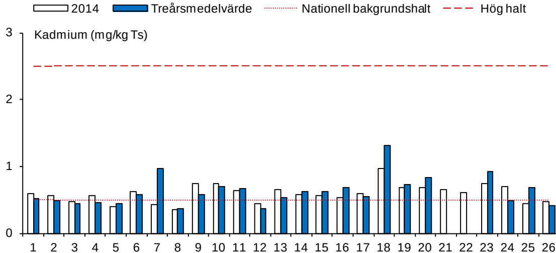
Figur 4. Halter av kadmium vid samtliga undersökta lokaler 2014 samt beräknade treårsmedelvärden. Halter över 2,5 mg/kg Ts klassas som höga (streckad linje). Den prickade linjen anger nationell bakgrundshalt (0,5 mg/kg Ts).
