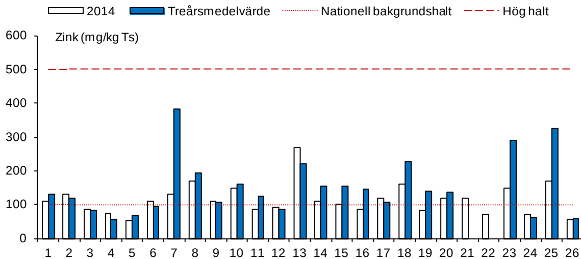
Figur 8. Halter av zink vid samtliga undersökta lokaler 2014 samt beräknade treårsmedelvärden. Halter över 500 mg/kg Ts klassas som höga (streckad linje). Den prickade linjen anger nationell bakgrundshalt (100 mg/kg Ts).
