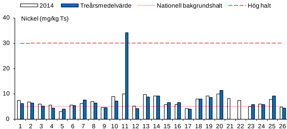
Figur 10. Halter av nickel vid samtliga undersökta lokaler 2014 samt beräknade treårsmedelvärden. Halter över 30 mg/kg Ts klassas som höga (streckad linje). Den prickade linjen anger nationell bakgrundshalt (5 mg/kg Ts).
