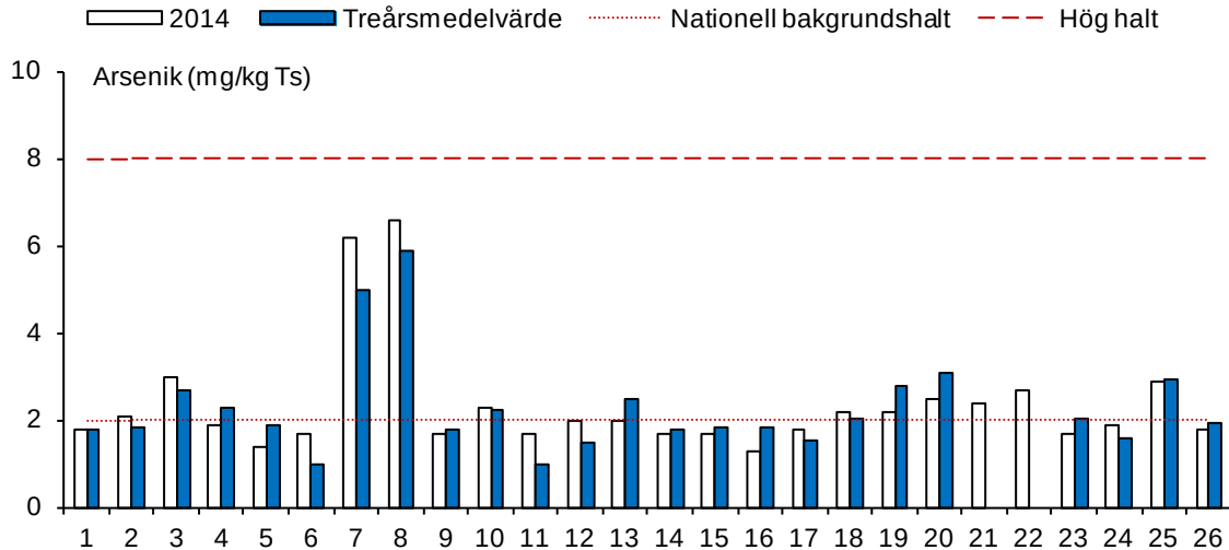
Figur 6. Halter av arsenik vid samtliga undersökta lokaler 2014 samt beräknade treårsmedelvärden. Halter över 8 mg/kg Ts klassas som höga (streckad linje). Den prickade linjen anger nationell bakgrundshalt (2 mg/kg Ts).
