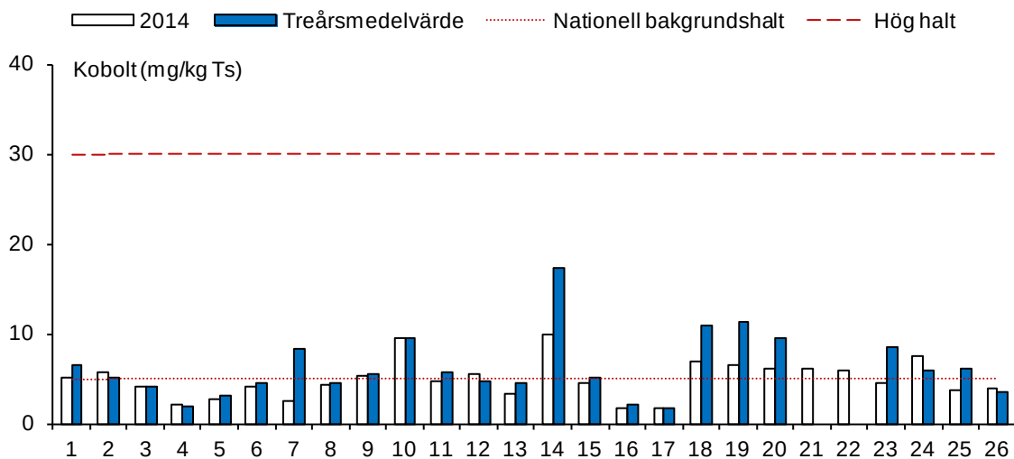
Figur 11. Halter av kobolt vid samtliga undersökta lokaler 2014 samt beräknade treårsmedelvärden. Halter över 30 mg/kg Ts klassas som höga (streckad linje). Den prickade linjen anger nationell bakgrundshalt (5 mg/kg Ts).
