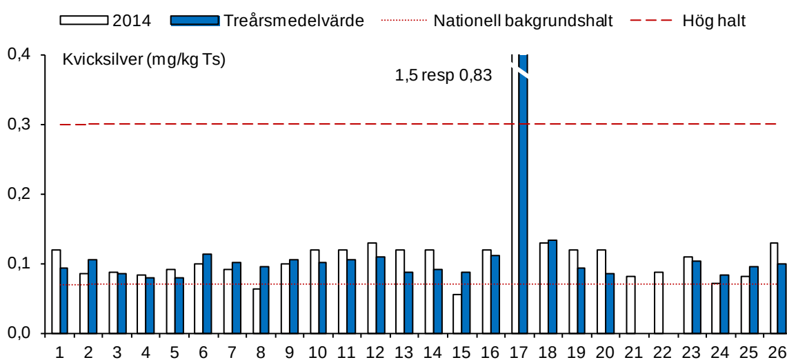
Figur 3. Halter av kvicksilver vid samtliga undersökta lokaler 2014 samt beräknade treårsmedelvärden. Halter över 0,3 mg/kg Ts klassas som höga (streckad linje). Den prickade linjen anger nationell bakgrundshalt (0,07 mg/kg Ts).
