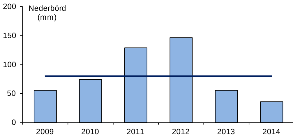
Figur 2. Medelnederbörd i Göteborg under september 2009-2014. Linjen anger normalvärden (1961-1990).
