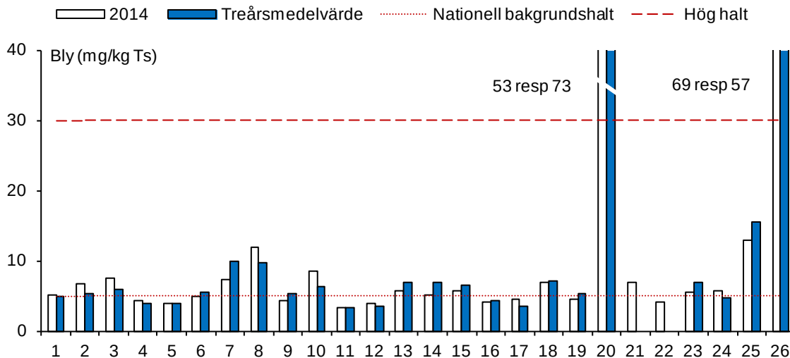
Figur 5. Halter av bly vid samtliga undersökta lokaler 2014 samt beräknade treårsmedelvärden. Halter över 30 mg/kg Ts klassas som höga (streckad linje). Den prickade linjen anger nationell bakgrundshalt (5 mg/kg Ts).
