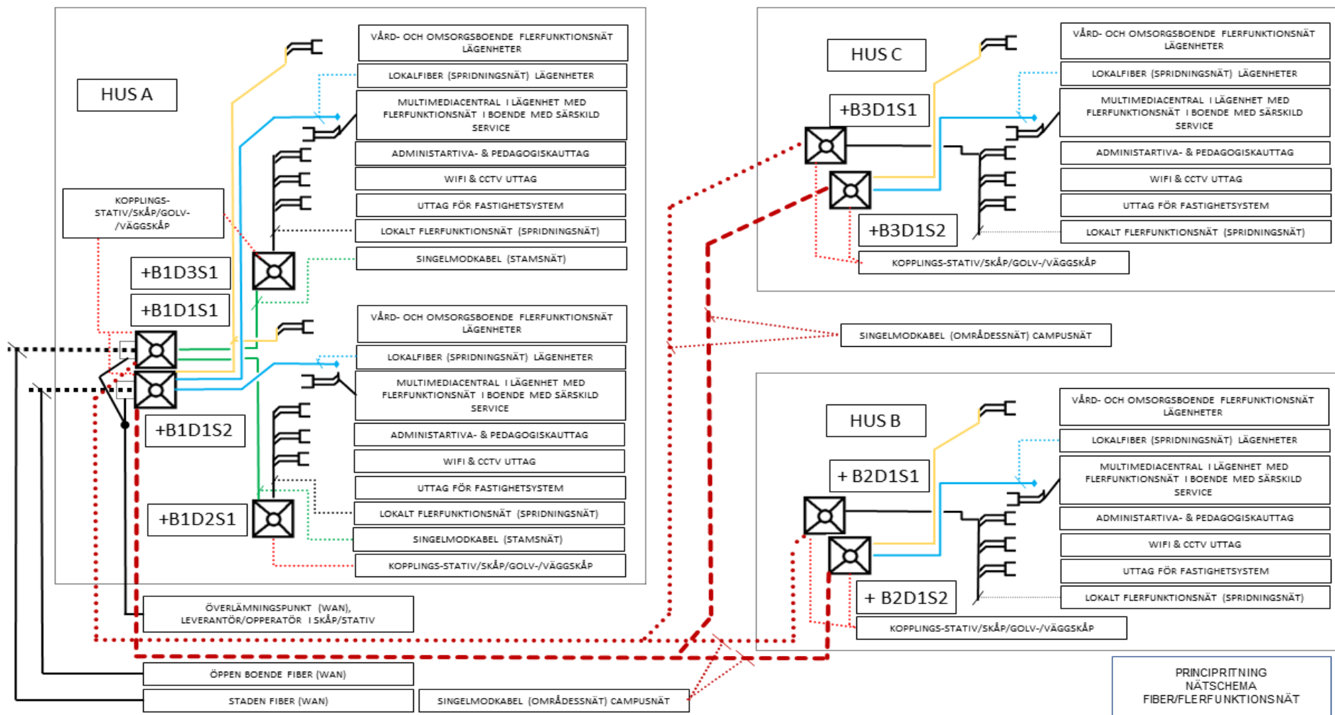
Figur 1 Nätschema för fiber- och datanät.
