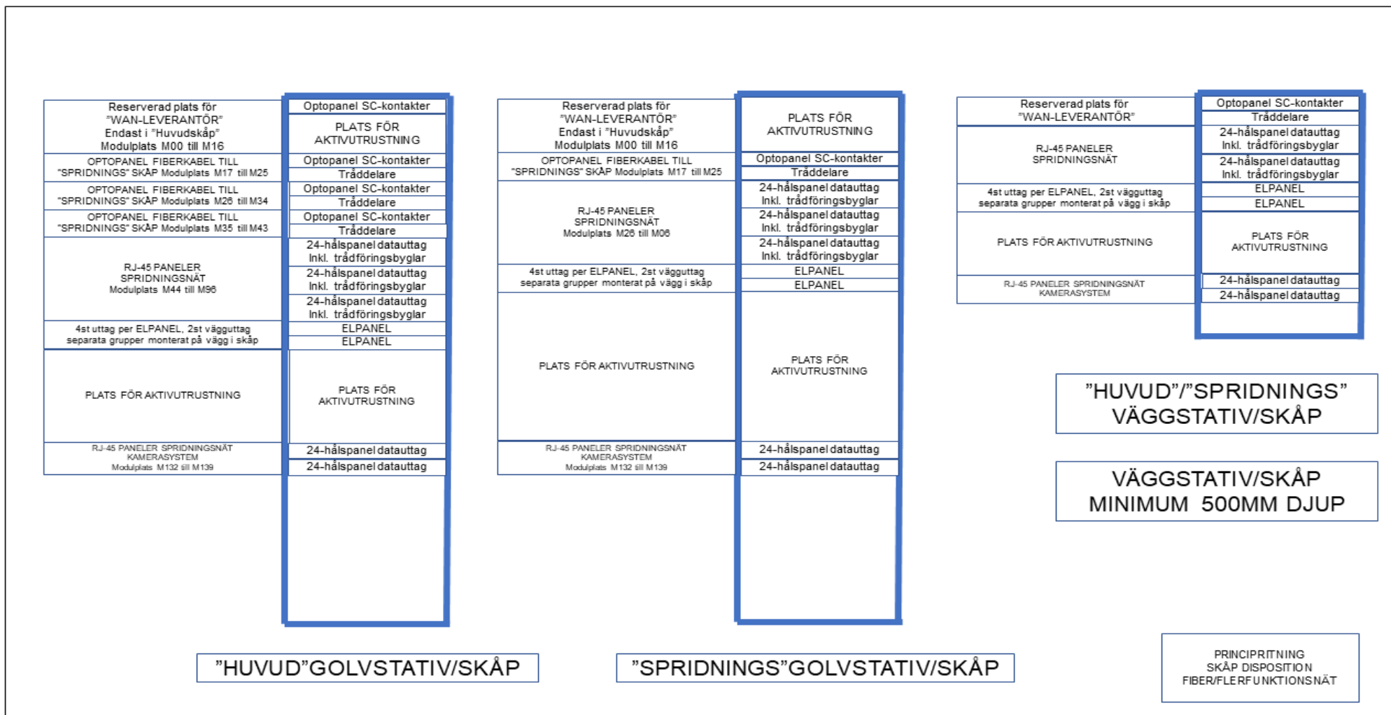
Figur 2 Disposition av stativ/skåp för fiber- och datanät.
