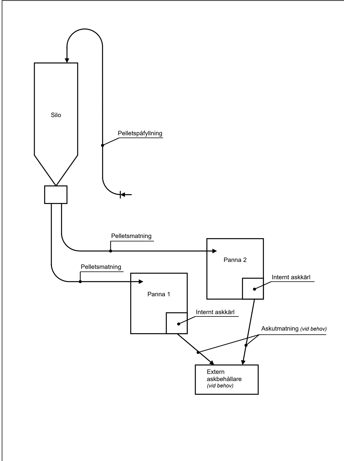
Figur 1. Systemuppbyggnad pannanläggning.
