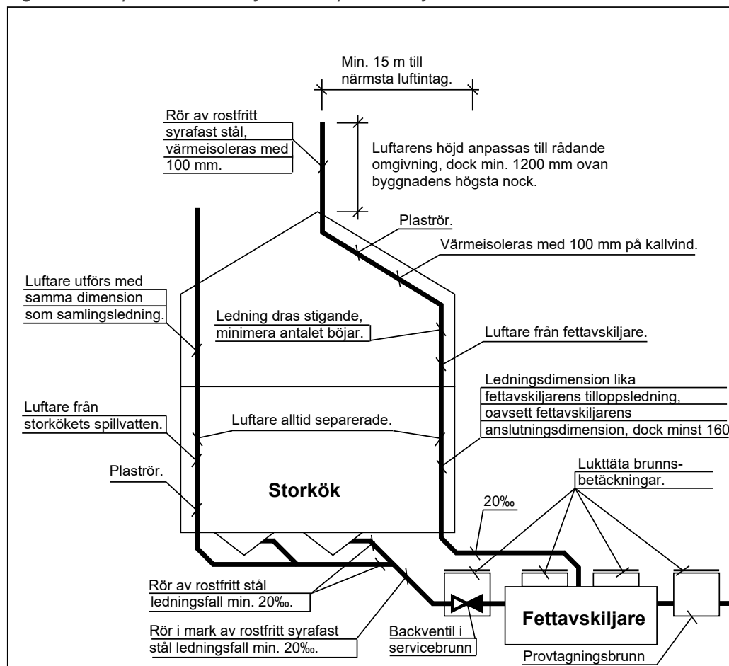
Figur 1. Principer för fettavskiljare och spillvattensystem från storkök.
