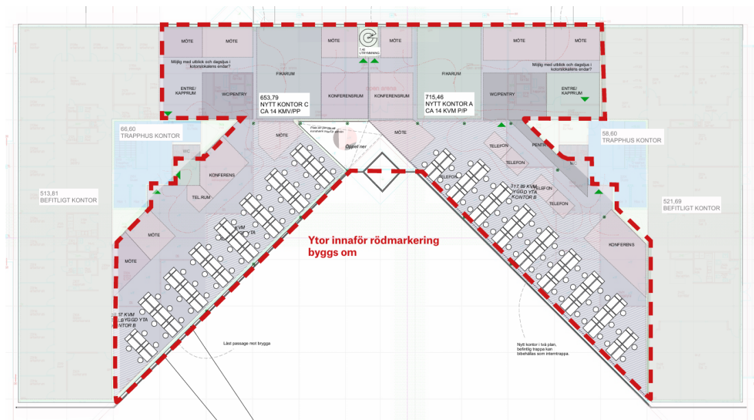
Figur 3 Plan 1, område med röd streckad linje ingår i förstudiekalkylen. Övriga lokaler är för närvarande uthyrda.
