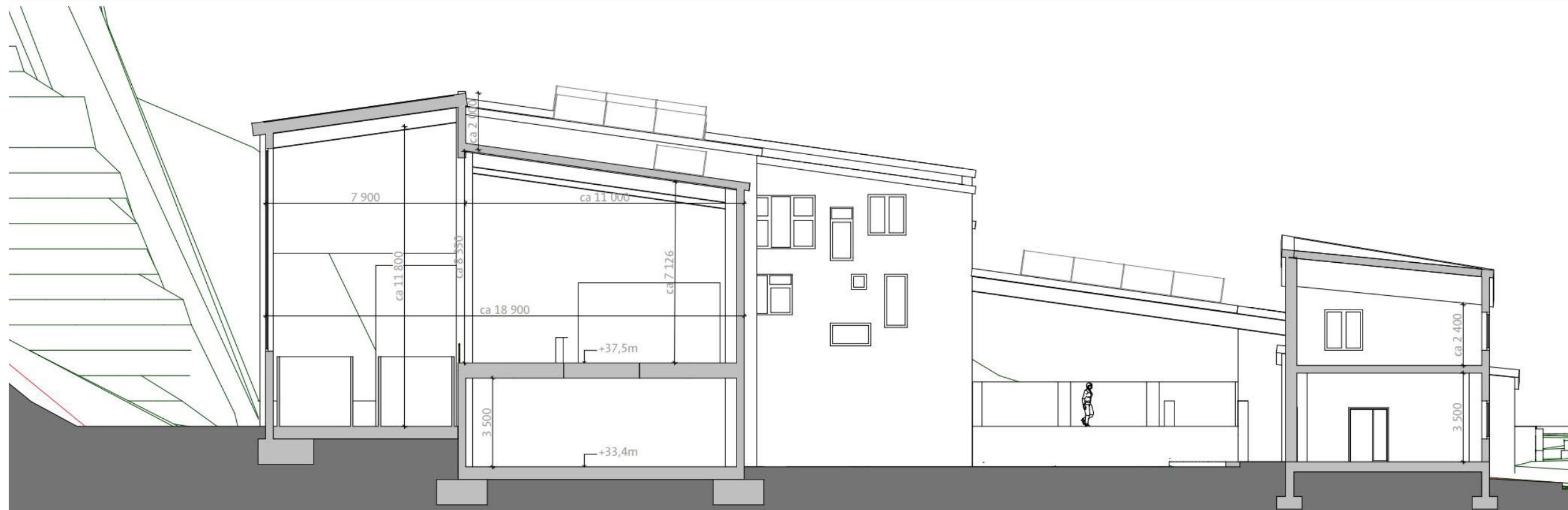
SEKTIONER A-A OCH B-B FÖR KRETSLOPPSPARKEN, TORSTENSSON ART & DESIGN AB 2022-06-16
