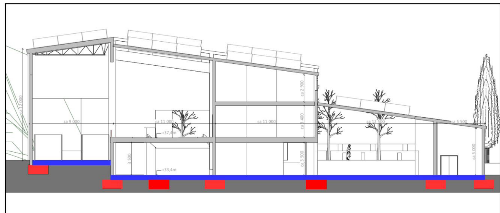
Figur 9 - Grundläggning den större byggnaden
