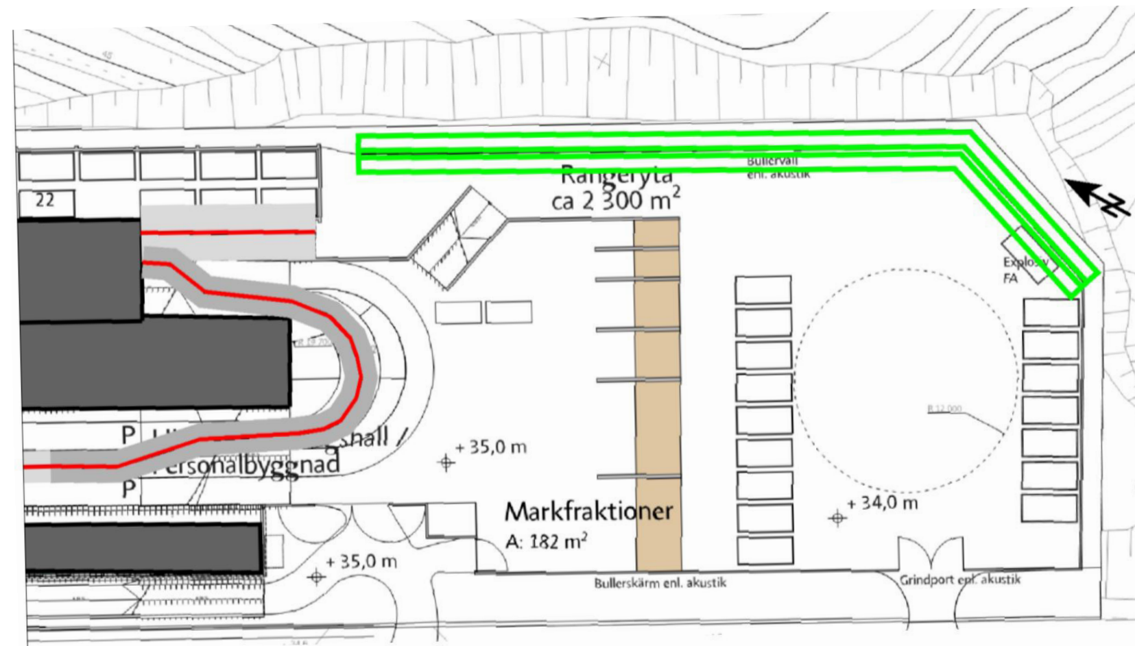
PLANERAD BULLERVALL MOT BERGET I GRÖNT, WSP AKUSTIK 2022-08-30
