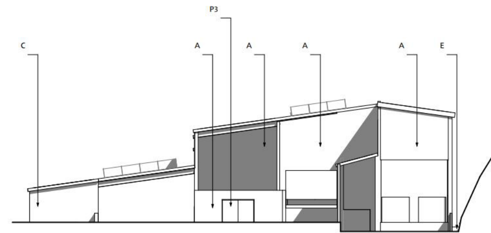
HUS 1 och HUS 2 - Fasad mot sydost 1:200
