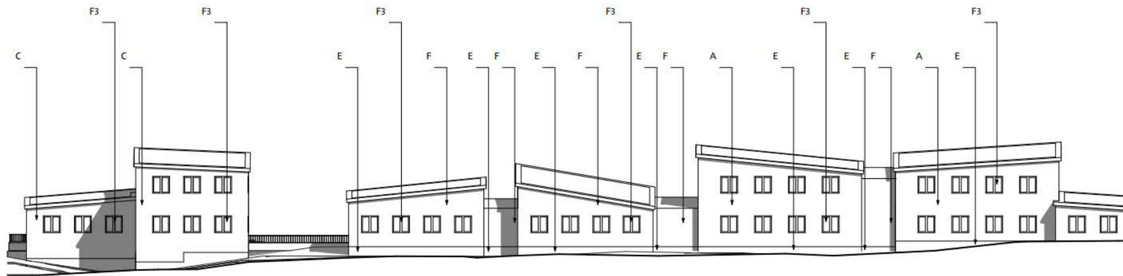
HUS 3, HUS 4, HUS 5 - Fasad mot sydväst 1:200
