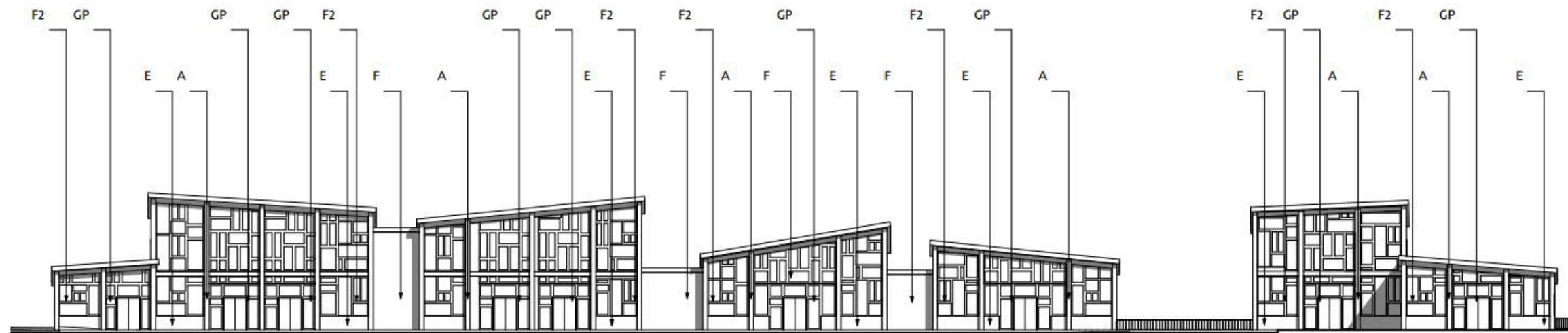
HUS 3, HUS 4 och HUS 5- Fasad mot nordost 1:200
