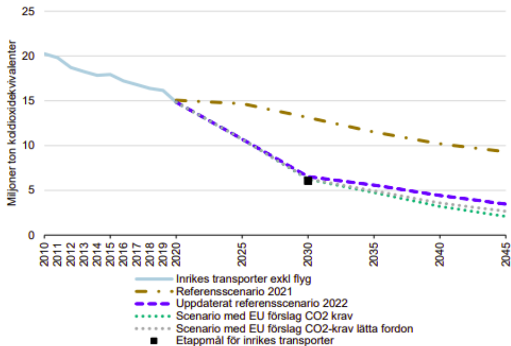
Figur 2.2. Utsläpp från inrikes transporter (exklusive inrikes flyg) till 2030, etappmålet till 2030, referensscenario 2021, uppdaterat referensscenario 2022, scenario med EU:s förslag till koldioxidkrav för lätta och tunga fordon samt scenario med koldioxidkrav endast för lätta fordon.
