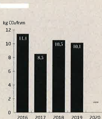
Totalt koldioxidutsläpp BOA/LOA**
