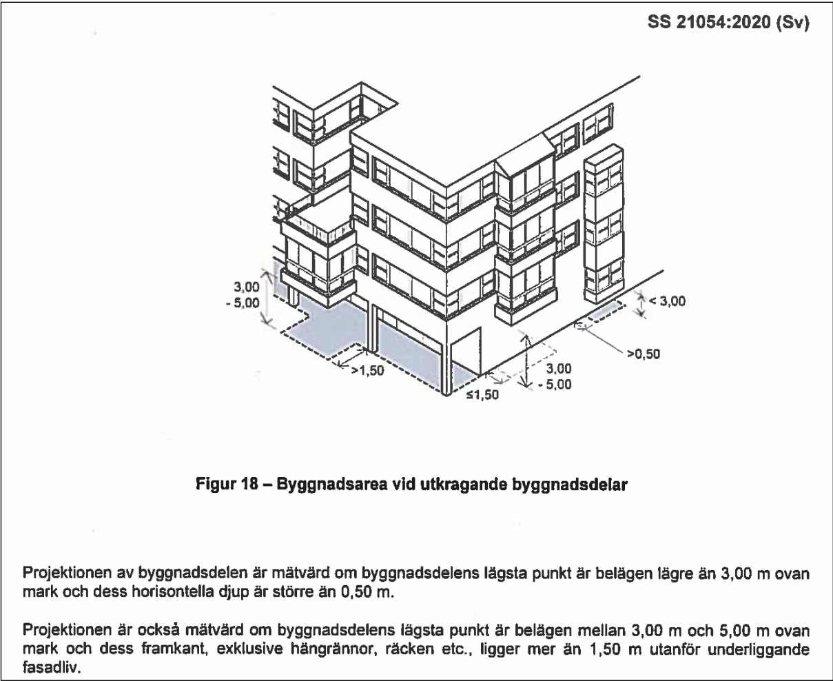
Illustration: utdrag ur SS 21054:2020 - Area och Volym anger förutsättningar för utkragande byggnadsdelar. SAMTALSUNDERLAG - 200601
