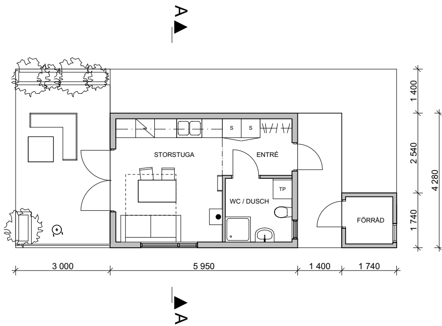
PLAN 1, SKALA 1:100
