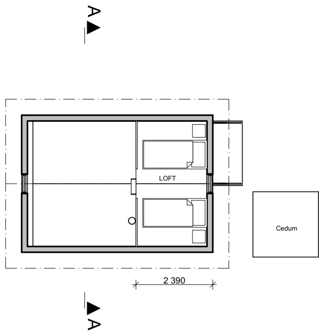
LOFT, SKALA 1:100
